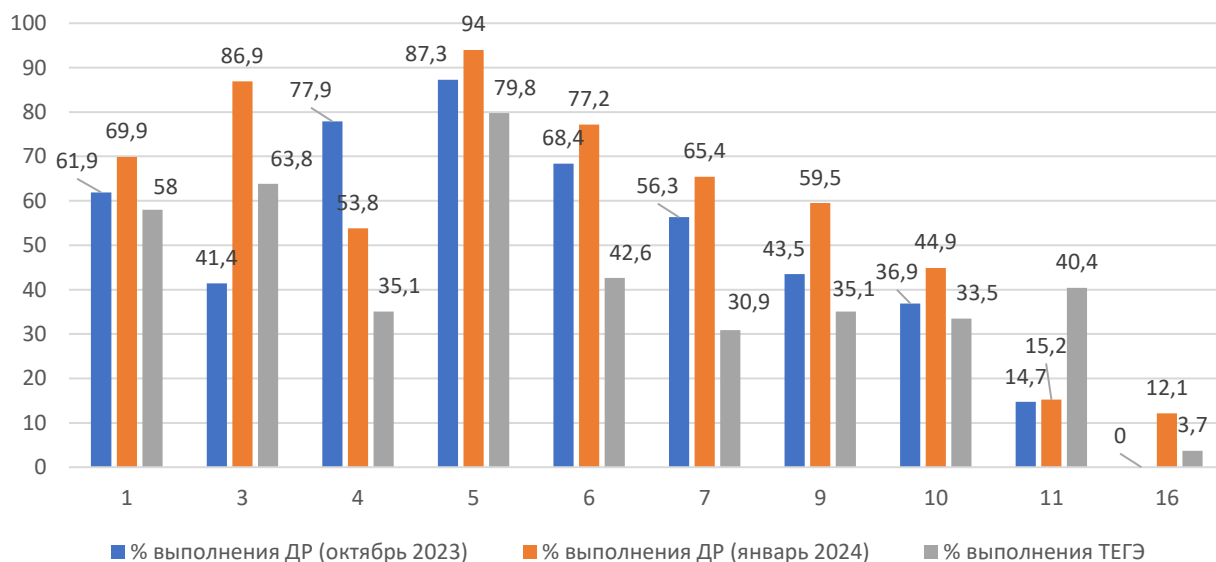
Рисунок 2. Сравнительный анализ выполнения заданий (%) по математике профильной 1
