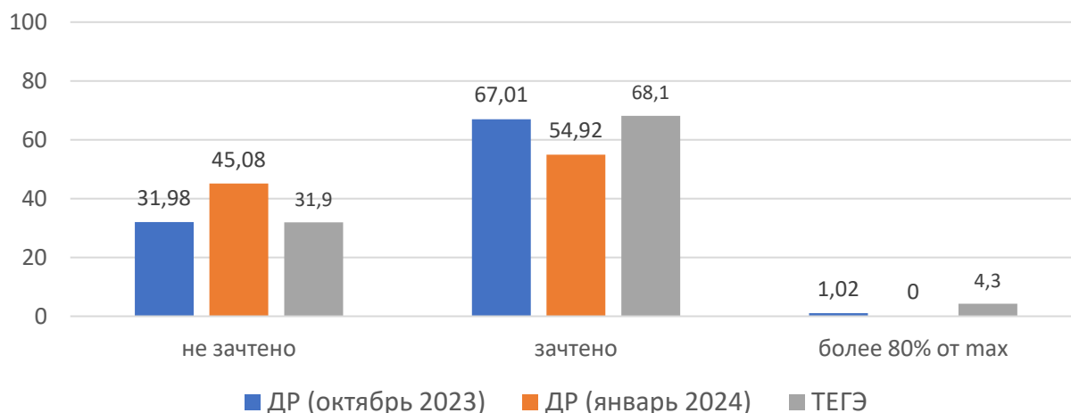
Рисунок 1. Основные результаты ДР по математике профильной
